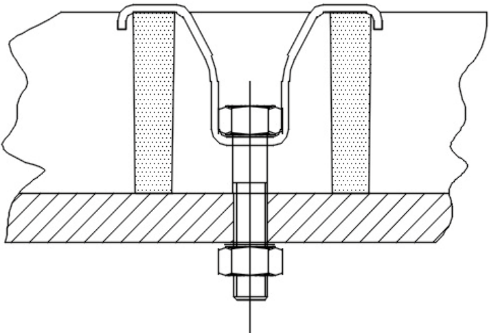
ESQUEMA TÍPICO DE FIJACIÓN
