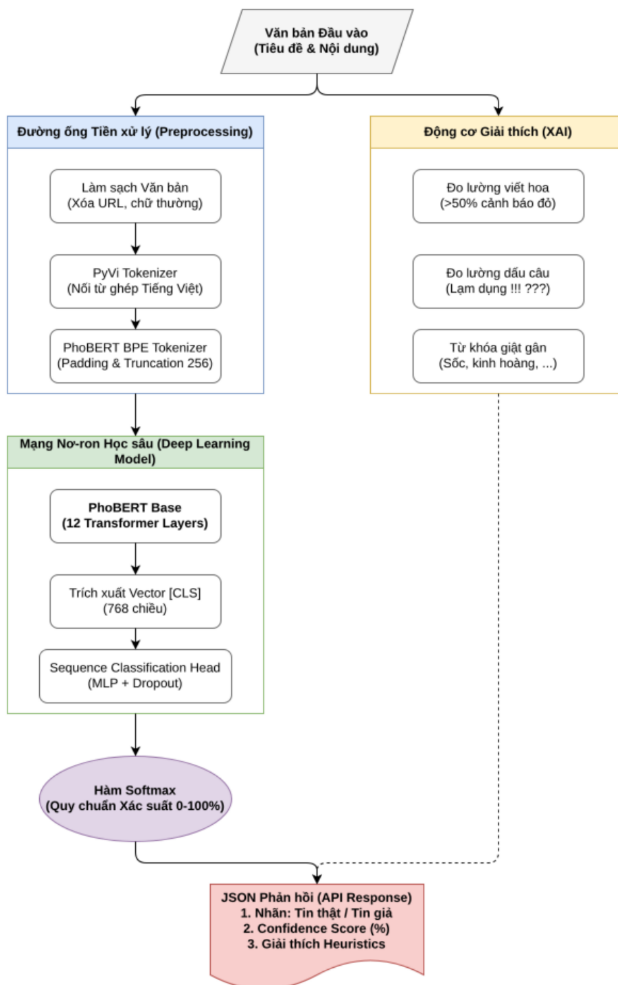
Hình 3.3: Lũy đồ xử lý thuật toán PhoBERT Sequence Classification
