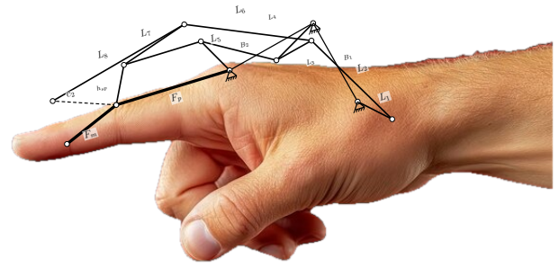
Figura 3. Mecanismo optimizado por la ED montado sobre un dedo simbólico, trazado a escala a partir de la cinemática real del modelo. La cadena de eslabones L_1-L_8 se sitúa sobre el dorso y las falanges F_p y F_m sobre las falanges proximal y medial; las juntas de revoluta se dibujan como círculos blancos, los apoyos fijos con achurado y la línea discontinua indica el balancín c_2 . Las dimensiones corresponden a la columna ED de la Tabla V (mecanismo después de optimizar); frente a la Fig. 1 se aprecia un diseño más compacto.
