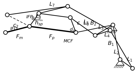
Figura 1. Diagrama de eslabones del modelo simplificado, generado con la cinemática real usando las dimensiones óptimas de la ED. Se etiquetan los parámetros de diseño: bancadas B_1 y B_2 , eslabones L_1 – L_8 , balancín c_2 , soporte c y desplazamientos h_{sp} y d_{sp} . Las falanges F_p y F_m tienen longitud fija ( |MCF-IFP| = 49 mm y |IFP-IFD| = 26 mm). El ángulo \theta_{aux_{fm}} orienta la falange medial respecto al balancín de la segunda etapa.
