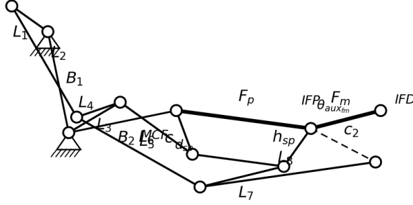
Figura 1. Diagrama de eslabones del modelo simplificado, generado con la cinemática real usando las dimensiones óptimas de la ED. Se etiquetan los parámetros de diseño: bancadas B_1 y B_2 , eslabones L_1 – L_8 , balancín c_2 , soporte c y desplazamientos h_{sp} y d_{sp} . Las falanges F_p y F_m tienen longitud fija ( |MCF-IFP| = 49 mm y |IFP-IFD| = 26 mm). El ángulo \theta_{aux\,fm} orienta la falange medial respecto al balancín de la segunda etapa.
