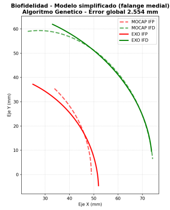
Figura 4. Biofidelidad de la solución del AG: las trayectorias de la IFP y la IFD acompañan a los puntos MOCAP; la IFD se ajusta con especial fidelidad.
