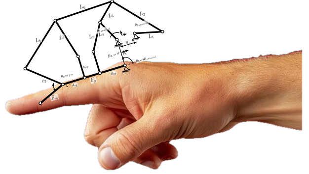
Figura 1. Mecanismo simplificado del exoesqueleto montado sobre un dedo simbólico: la cadena de eslabones L_1 – L_8 se sitúa sobre el dorso de la mano y las falanges F_p y F_m se alinean con las falanges proximal y medial del dedo. Las dimensiones de los eslabones representadas corresponden al mecanismo antes de optimizar .
