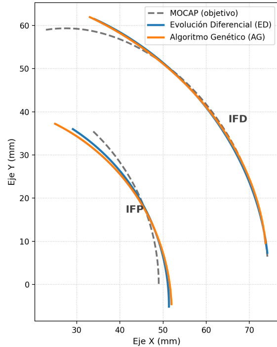
Figura 4. Biofidelidad de las trayectorias: curvas simuladas de la IFP y la IFD para la ED y el AG, superpuestas a los puntos MOCAP (objetivo) del agarre de pinza fina.
