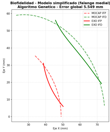
Figura 4. Biofidelidad de la solución del AG: la trayectoria de la IFD se aleja de los puntos MOCAP, en concordancia con su mayor error.
