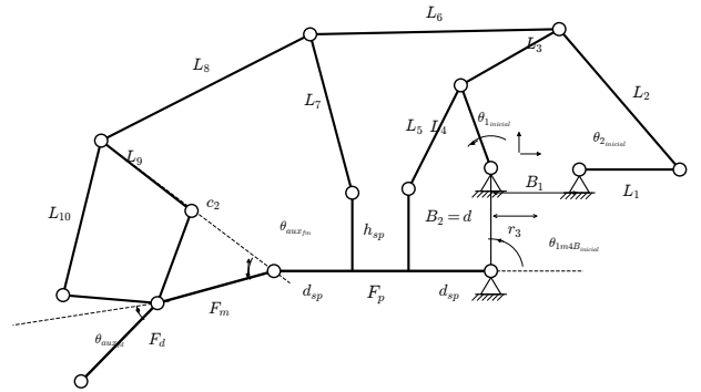
Figura 1. Esquema del mecanismo completo del exoesqueleto. La cadena de eslabones L_1 – L_{10} se ubica sobre el dorso del dedo, mientras que las falanges proximal F_p , medial F_m y distal F_d forman la línea inferior. Se indican las bancadas B_1 y B_2 = d , los balancines c_2 , las cotas r_3 , h_{sp} y d_{sp} , y los ángulos de entrada \theta_{1\text{inicial}} , \theta_{2\text{inicial}} y \theta_{1m4B\text{inicial}} . Los ángulos \theta_{auxfm} y \theta_{auxfd} orientan las falanges medial y distal respecto a los balancines de sus etapas. El modelo simplificado empleado en este trabajo corresponde a esta misma cadena hasta la falange medial ( L_1 – L_8 ). El esquema es ilustrativo y no está dibujado a escala.
