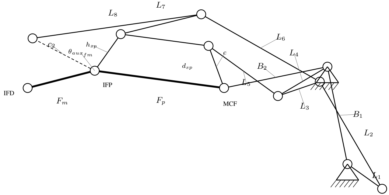
Figura 3. Diagrama de eslabones del mecanismo optimizado por la ED, trazado a escala a partir de la cinemática real del modelo (pose representativa a mitad del barrido de la manivela). Las juntas de revoluta se dibujan como círculos blancos y los apoyos fijos con achurado; la línea discontinua indica el balancín c_2 y las líneas gruesas, las falanges F_p y F_m . Las dimensiones de la cadena L_1-L_8 , las bancadas B_1 y B_2 y el balancín c_2 corresponden a la columna ED de la Tabla V.
