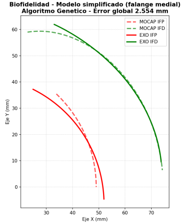
Figura 5. Biofidelidad de la solución del AG: las trayectorias de la IFP y la IFD siguen a los puntos MOCAP.
