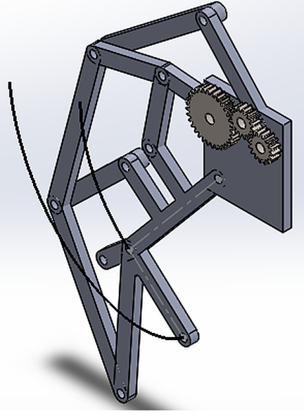
Figura 2. Modelo 3D del mecanismo de exoesqueleto antes de la optimización, al final de su recorrido. Las curvas trazadas muestran las trayectorias que siguen las articulaciones IFP e IFD durante el barrido completo de la manivela de entrada; estas rutas de trazo constituyen el objetivo de ajuste para la síntesis dimensional.
