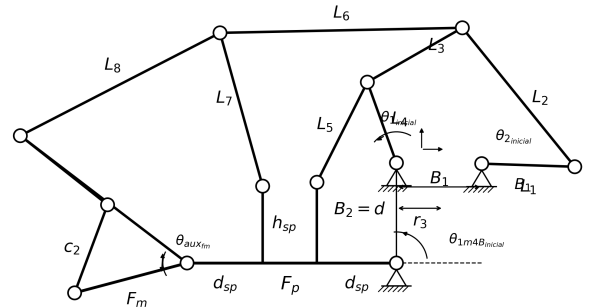
Figura 1. Esquema del mecanismo del modelo simplificado. La cadena de eslabones L_1 – L_8 se ubica sobre el dorso del dedo, mientras que las falanges proximal F_p y medial F_m forman la línea inferior. Se indican las bancadas B_1 y B_2 = d , el balancín c_2 , las cotas r_3 , h_{sp} y d_{sp} , y los ángulos de entrada \theta_{1inicial} , \theta_{2inicial} y \theta_{1m4Binicial} . El ángulo \theta_{auxfm} orienta la falange medial respecto al balancín de la segunda etapa. El esquema es ilustrativo y no está dibujado a escala.
