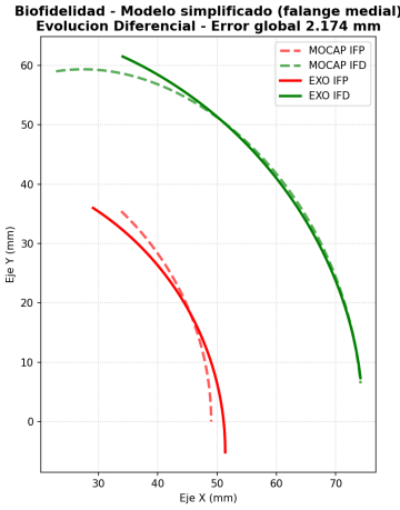
Figura 3. Biofidelidad de la solución de la ED: trayectorias simuladas (IFP e IFD) superpuestas a los puntos MOCAP.
