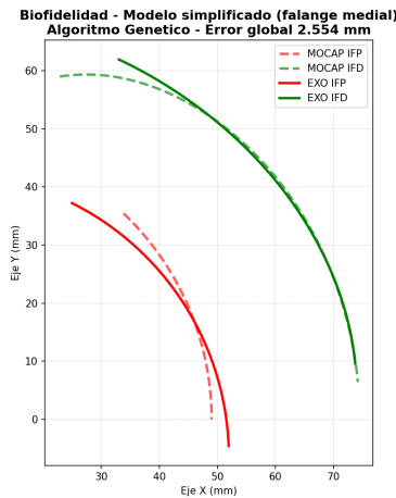
Figura 4. Biofidelidad de la solución del AG: las trayectorias de la IFP y la IFD acompañan a los puntos MOCAP; la IFD se ajusta con especial fidelidad.
