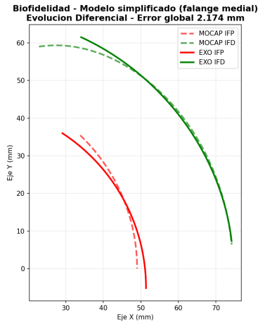
Figura 4. Biofidelidad de la solución de la ED: trayectorias simuladas (IFP e IFD) superpuestas a los puntos MOCAP.
