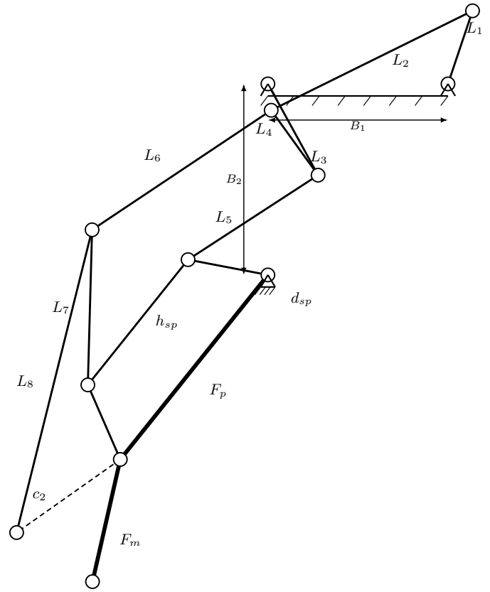
Figura 3. Diagrama de eslabones del mecanismo optimizado por la ED, trazado a partir de la cinemática real del modelo. Las bancadas B_1 y B_2 se indican como cotas (no son eslabones físicos); la línea discontinua es el balancín c_2 y las líneas gruesas son las falanges F_p y F_m . Las dimensiones de la cadena L_1-L_8 corresponden a la columna ED de la Tabla V (mecanismo después de optimizar).
