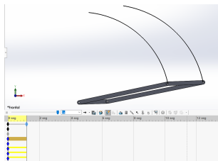
Figura: Estudio de movimiento
