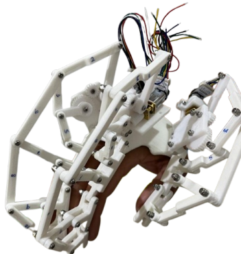
Figure: Mecanismo construido
