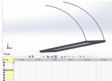
Figure: Mecanismo de 4 barras
