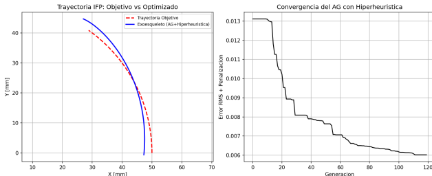
Figure: Resultado del AG con hiperheurística para la articulación IFP
