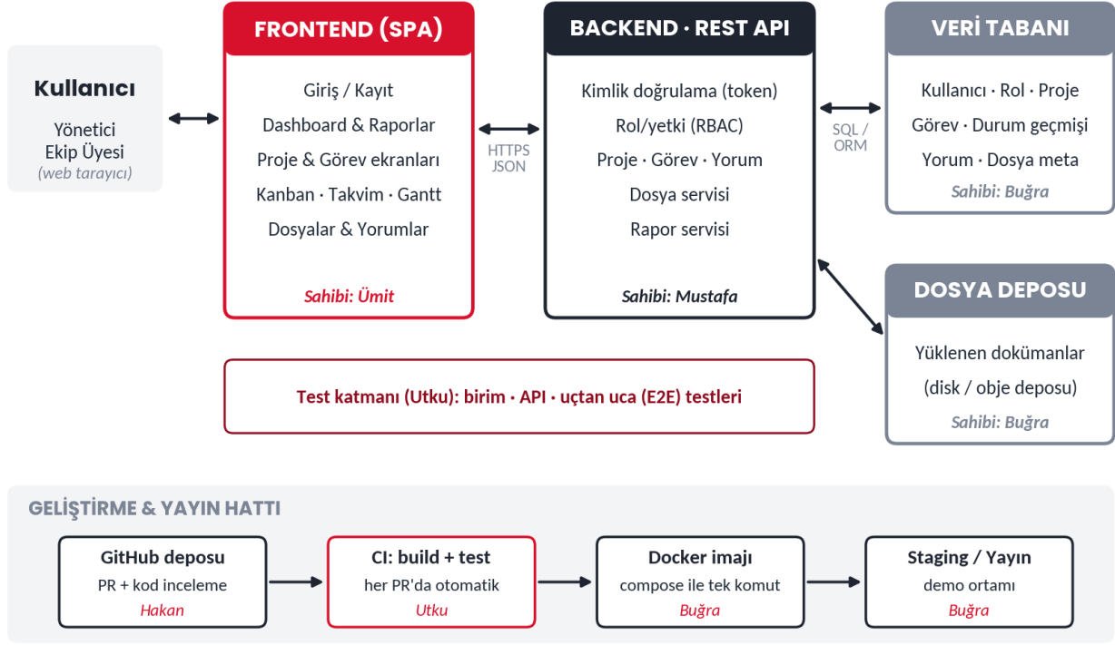
Şekil 8 · Üç katmanlı mimari ve geliştirme/yayın hattı
