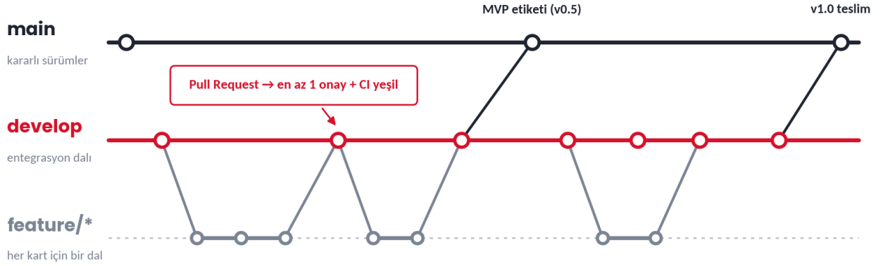
Şekil 5 - main / develop / feature dal modeli
