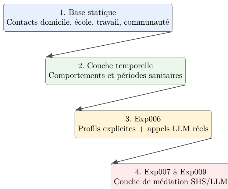
FIGURE 1 – Logique générale du manuscrit.
