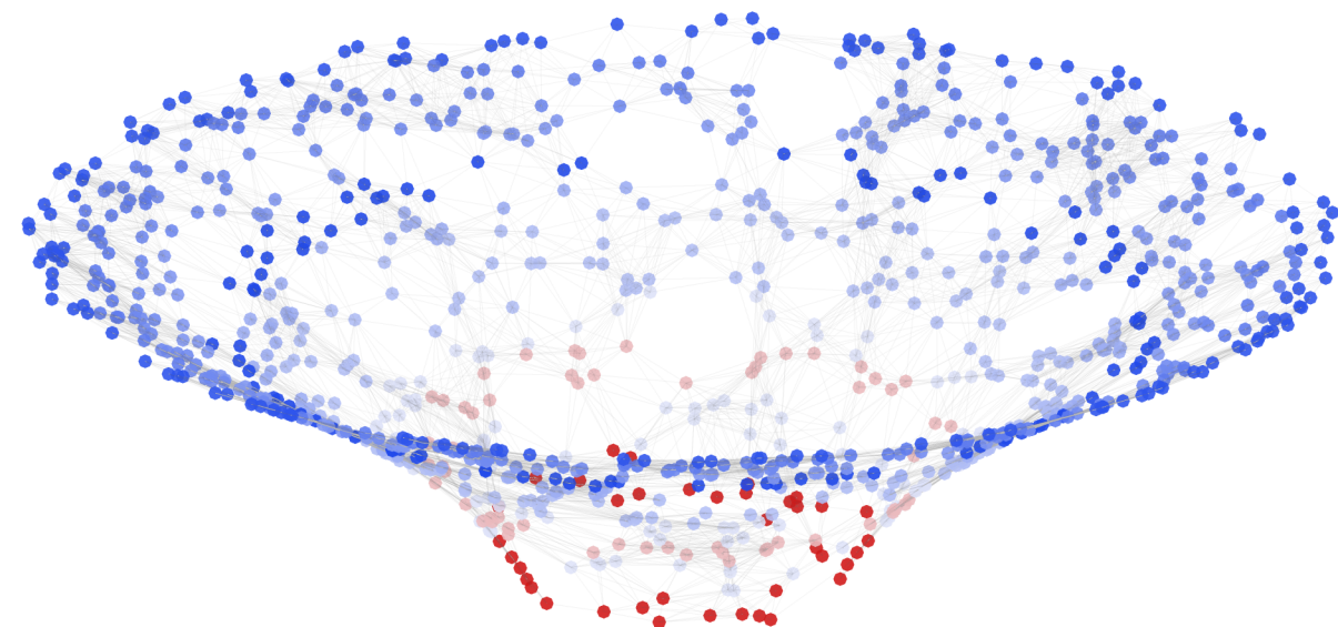
Schwarzschild / Flamm
