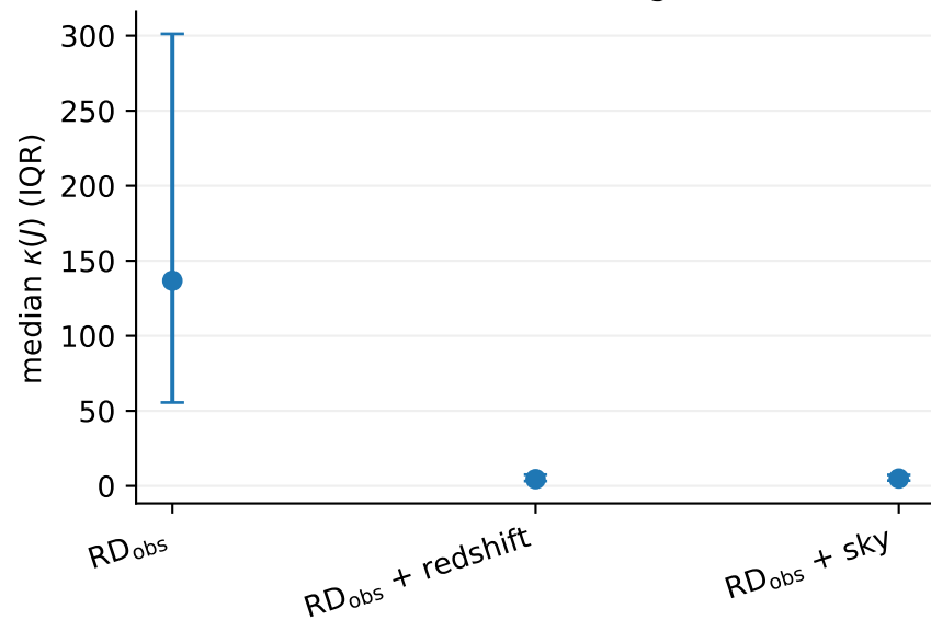
B. Conditioning
