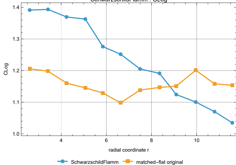
SchwarzschildFlamm : CLog
