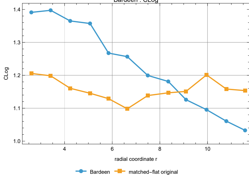
Bardeen : CLog
