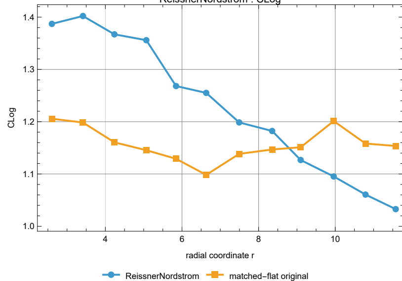
ReissnerNordstrom : CLog
