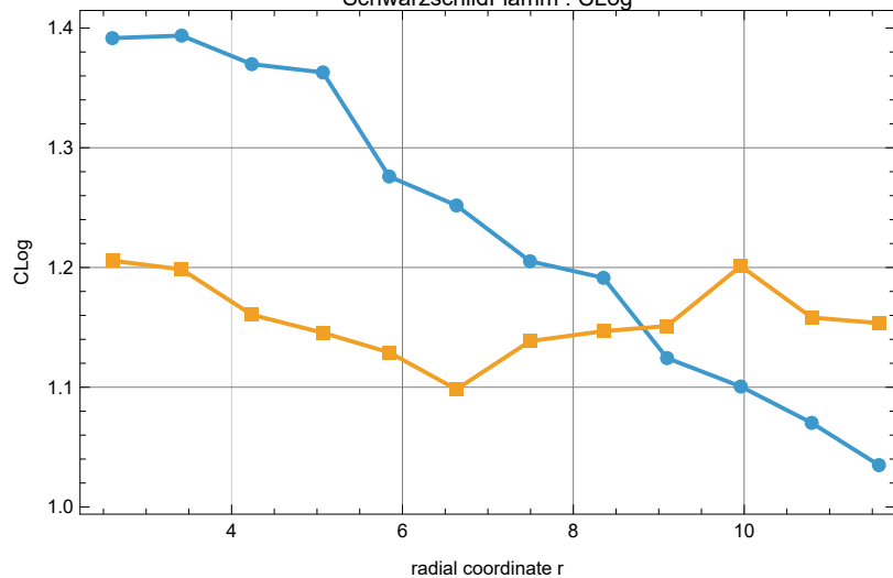
SchwarzschildFlamm : CLog
