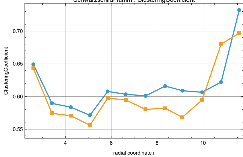
SchwarzschildFlamm : ClusteringCoefficient
