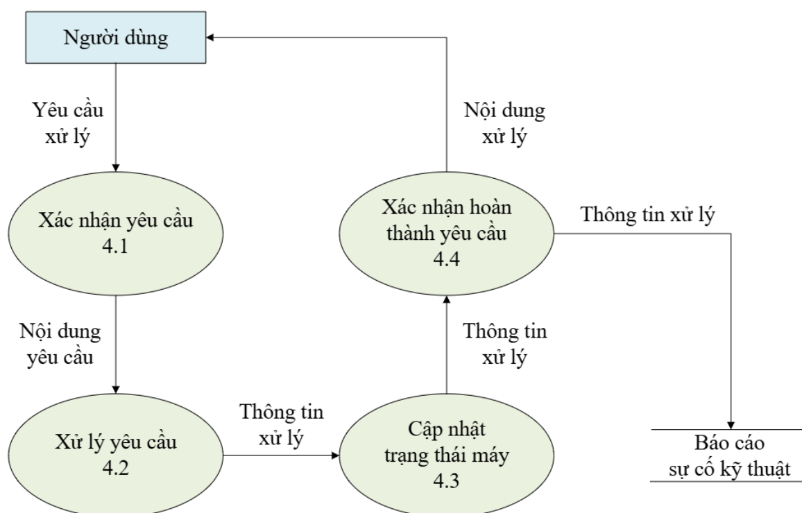
Hình 3.34: Sơ đồ DFD mức 1 - Xử lý hỗ trợ kỹ thuật
