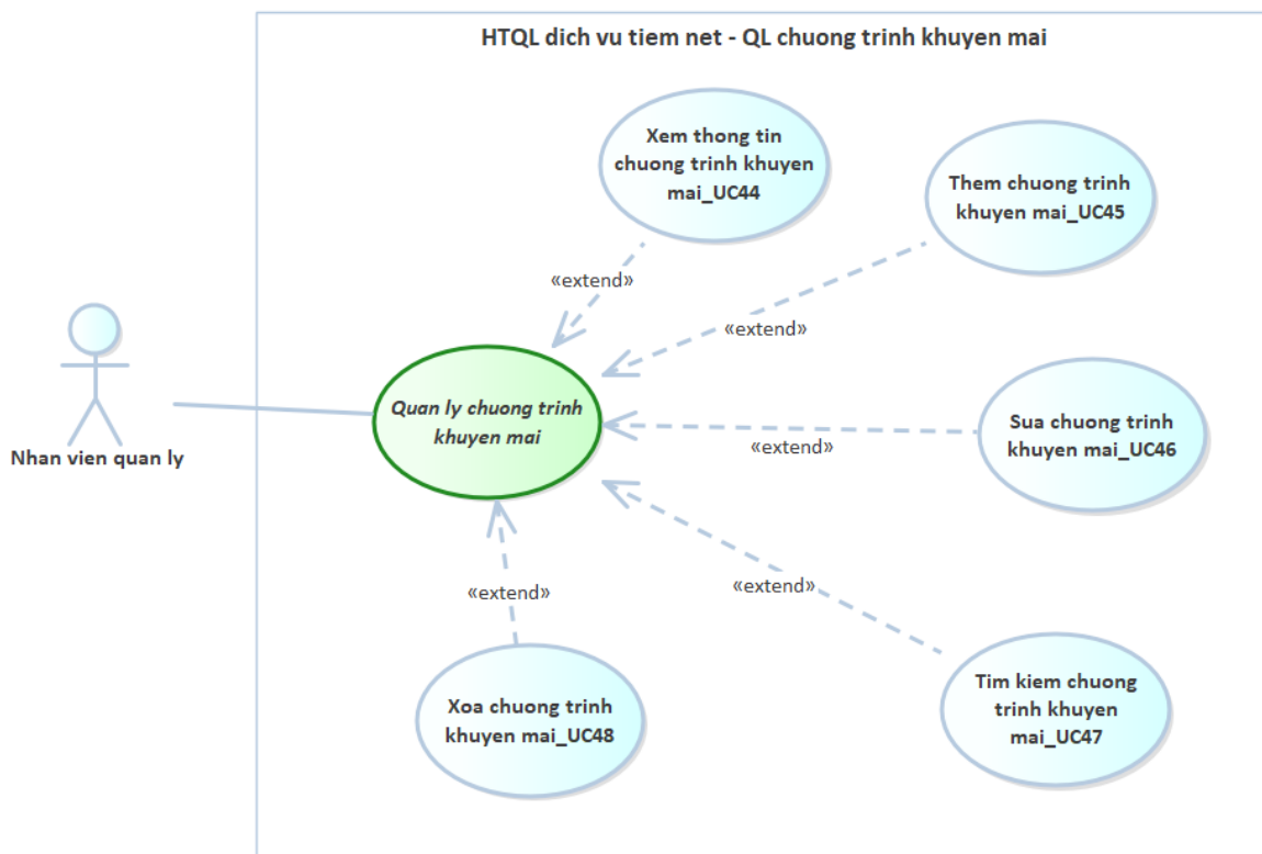
Hình 2.8: Sơ đồ use case mức chi tiết - QL chương trình khuyến mãi
