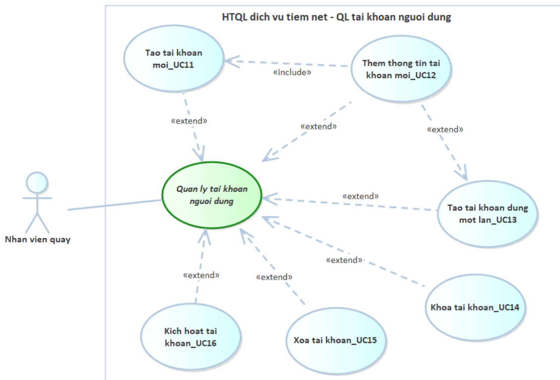
Hình 2.3: Sơ đồ use case mức chi tiết - QL tài khoản người dùng
