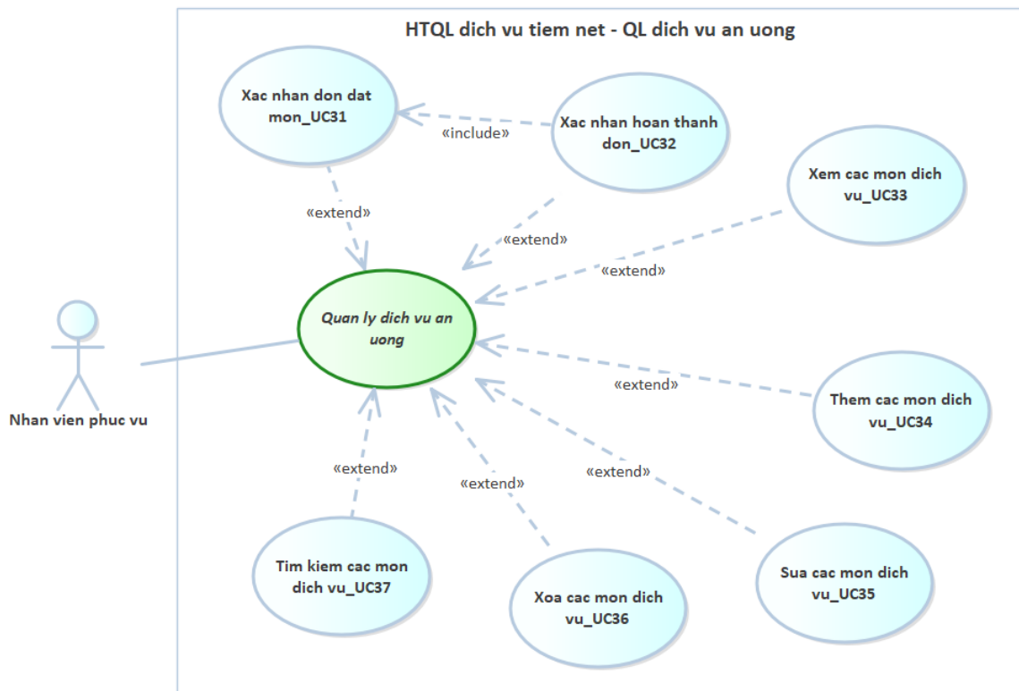
Hình 2.6: Sơ đồ use case mức chi tiết - QL dịch vụ ăn uống
