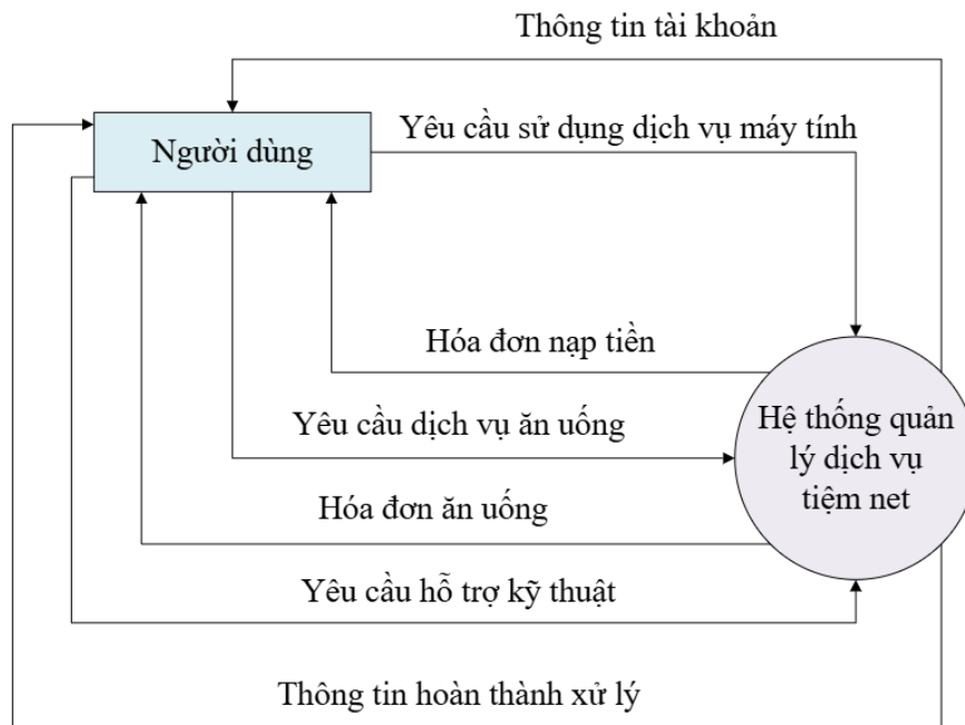
Hình 3.29: Sơ đồ DFD mức ngữ cảnh
