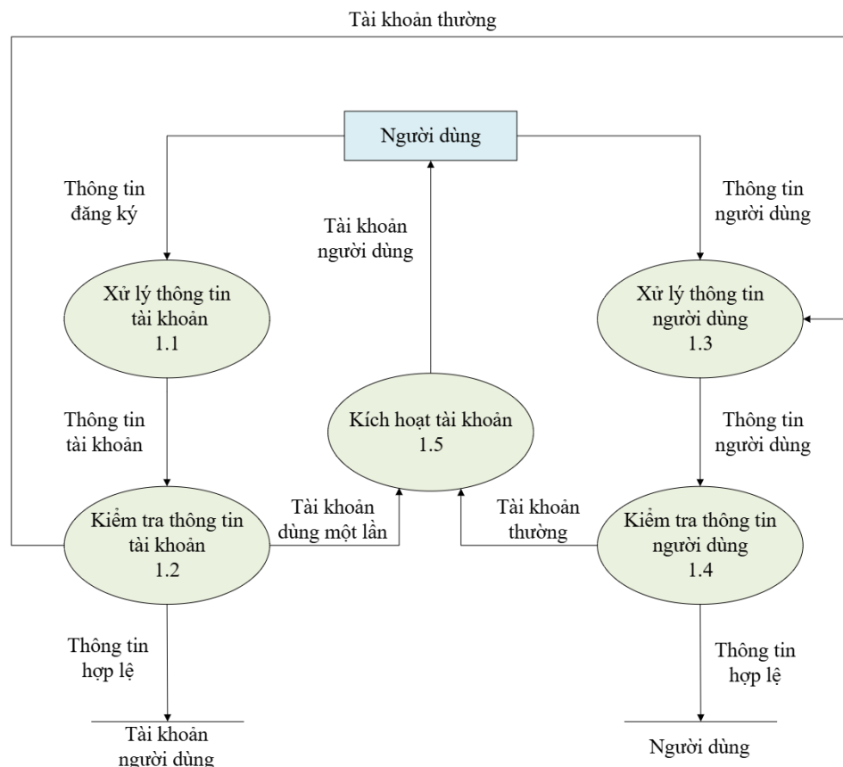
Hình 3.31: Sơ đồ DFD mức 1 - đăng ký tài khoản
