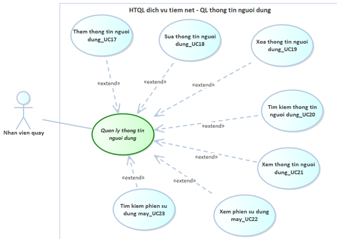
Hình 2.4: Sơ đồ use case mức chi tiết - QL thông tin người dùng
