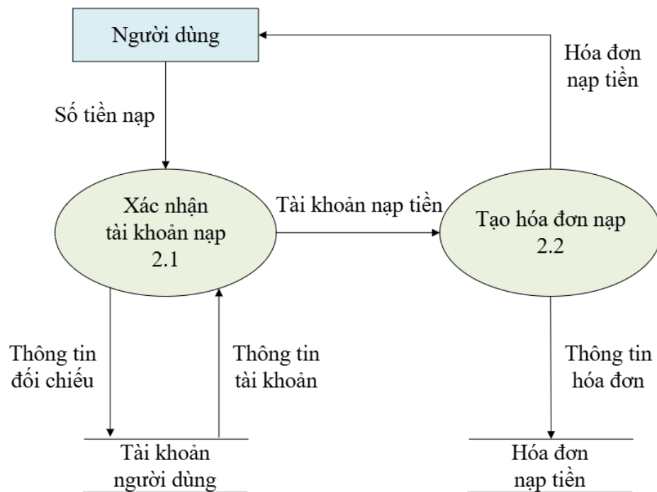
Hình 3.32: Sơ đồ DFD mức 1 - nạp tiền
