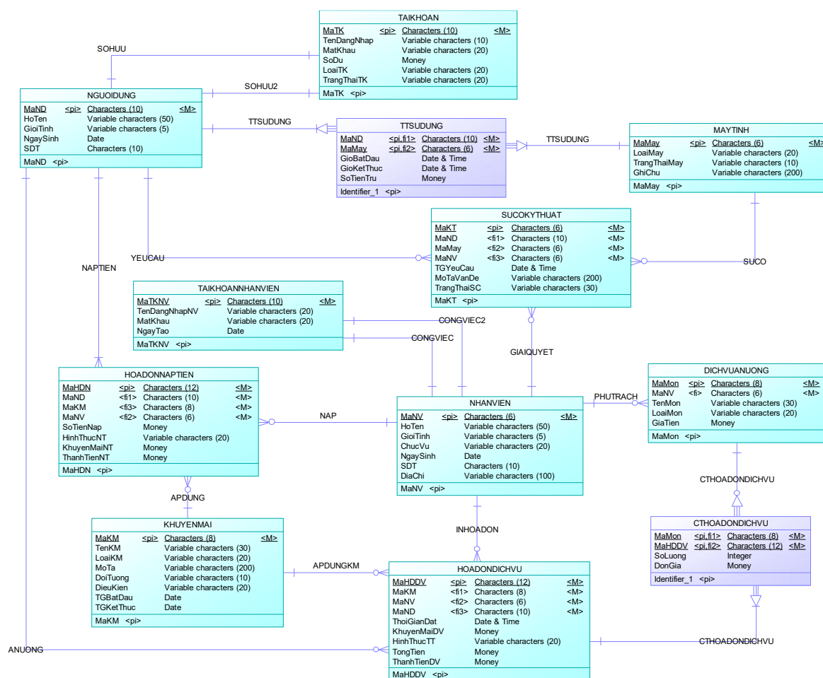
Hình 3.2: Mô hình mức logic
