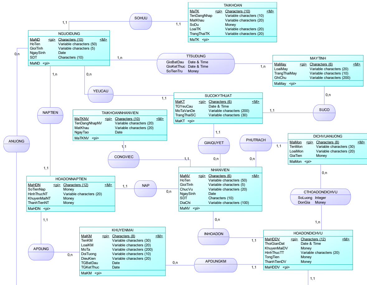
Hình 3.1: Mô hình mức quan niệm
