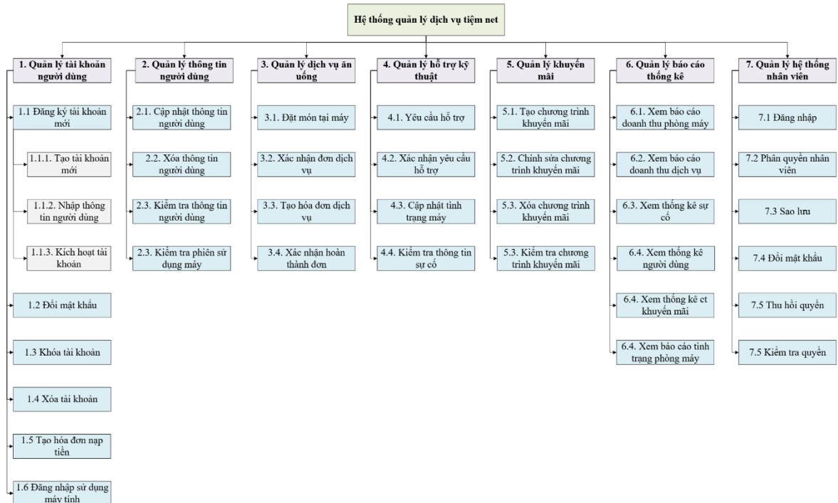
Hình 3.28: Mô hình phân rã chức năng (BFD)
