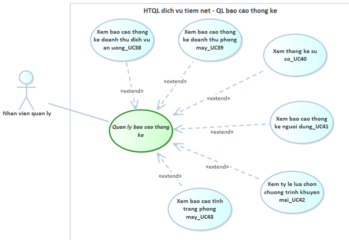
Hình 2.7: Sơ đồ use case mức chi tiết - QL báo cáo thống kê
