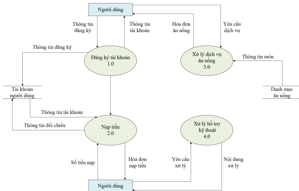
Hình 3.30: Sơ đồ DFD mức 0
