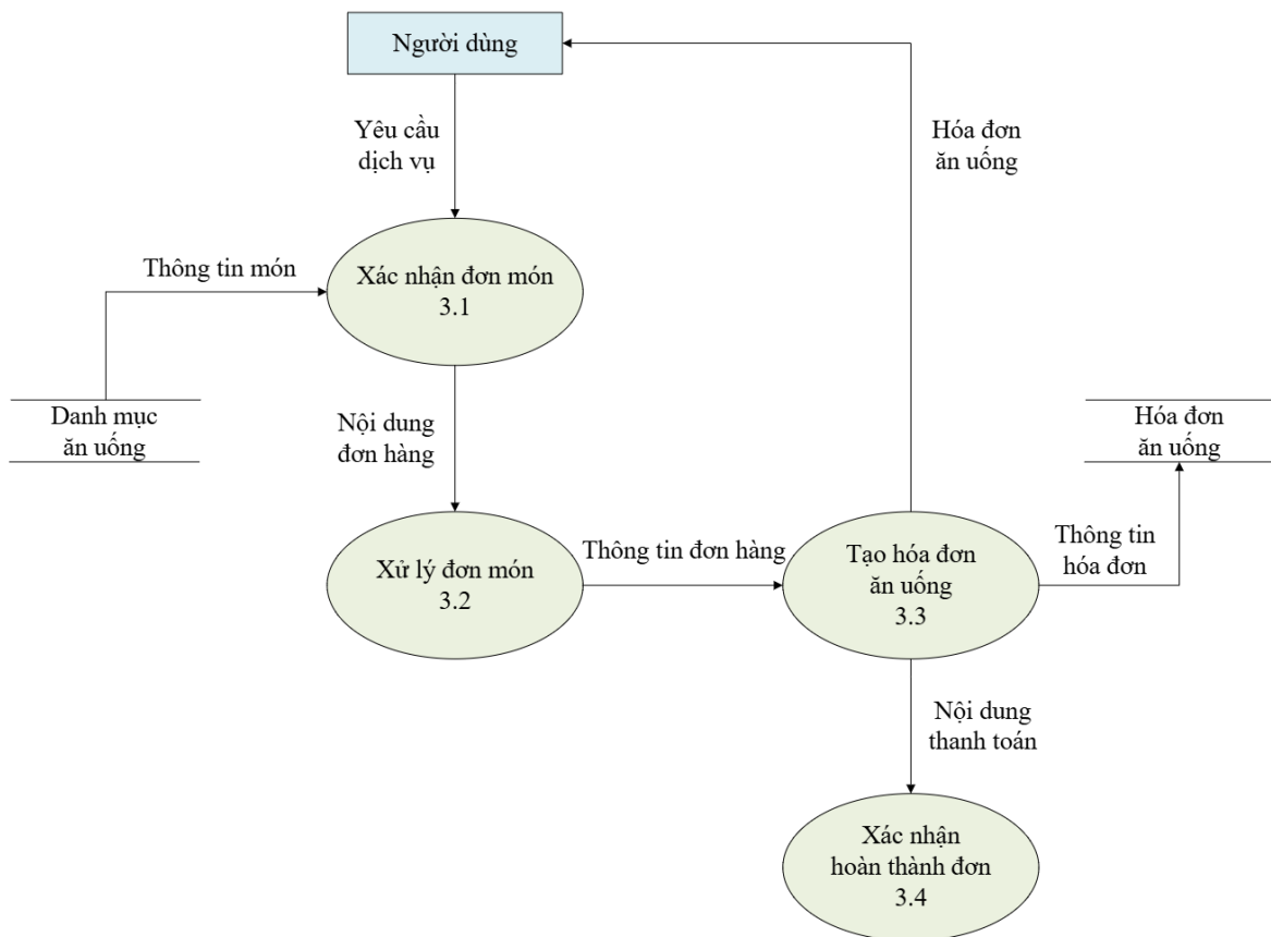
Hình 3.33: Sơ đồ DFD mức 1 - Xử lý dịch vụ ăn uống
