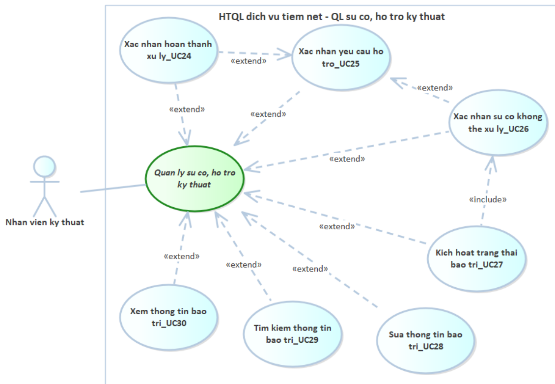
Hình 2.5: Sơ đồ use case mức chi tiết - QL sự cố, hỗ trợ kỹ thuật
