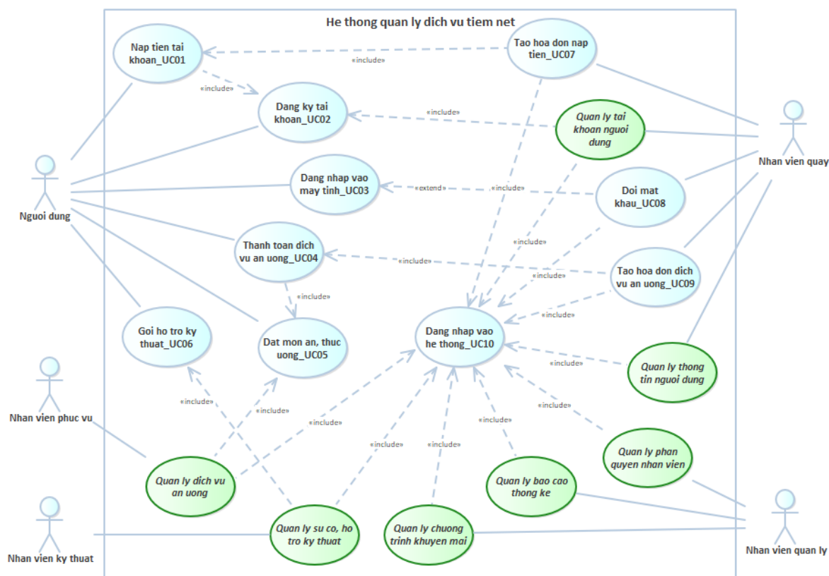
Hình 2.2: Sơ đồ use case mức tổng thể
