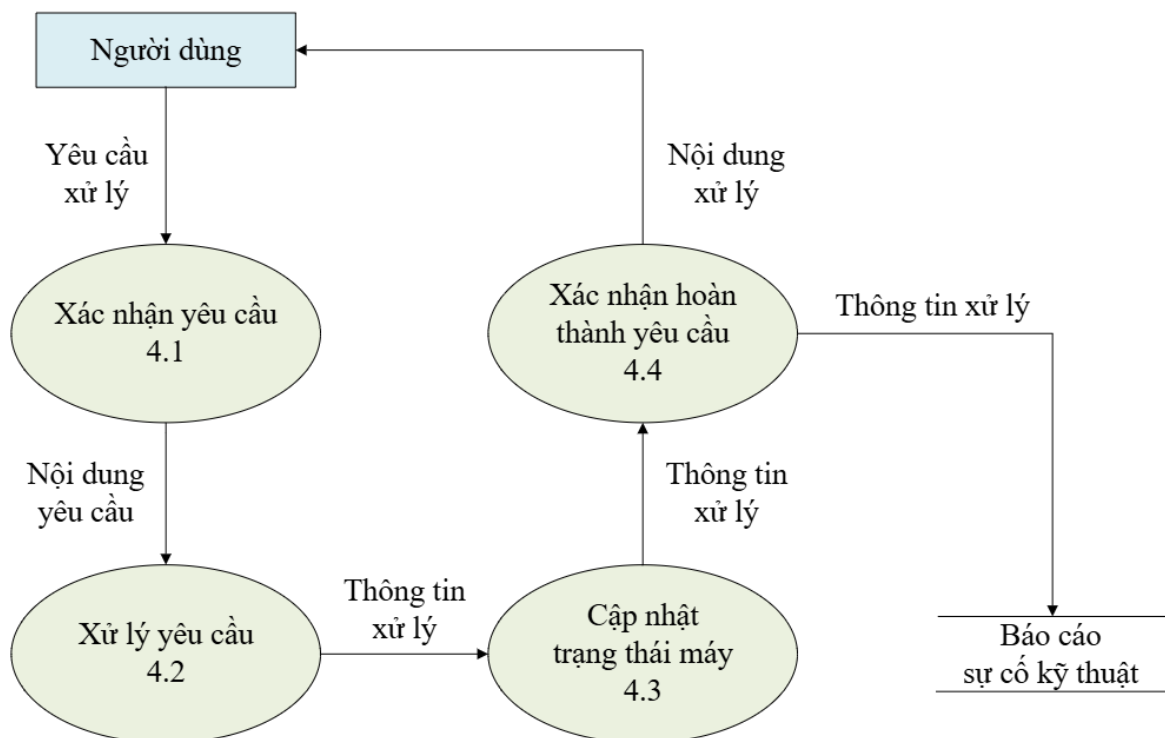
Hình 3.7: Sơ đồ DFD mức 1 - Xử lý hỗ trợ kỹ thuật
