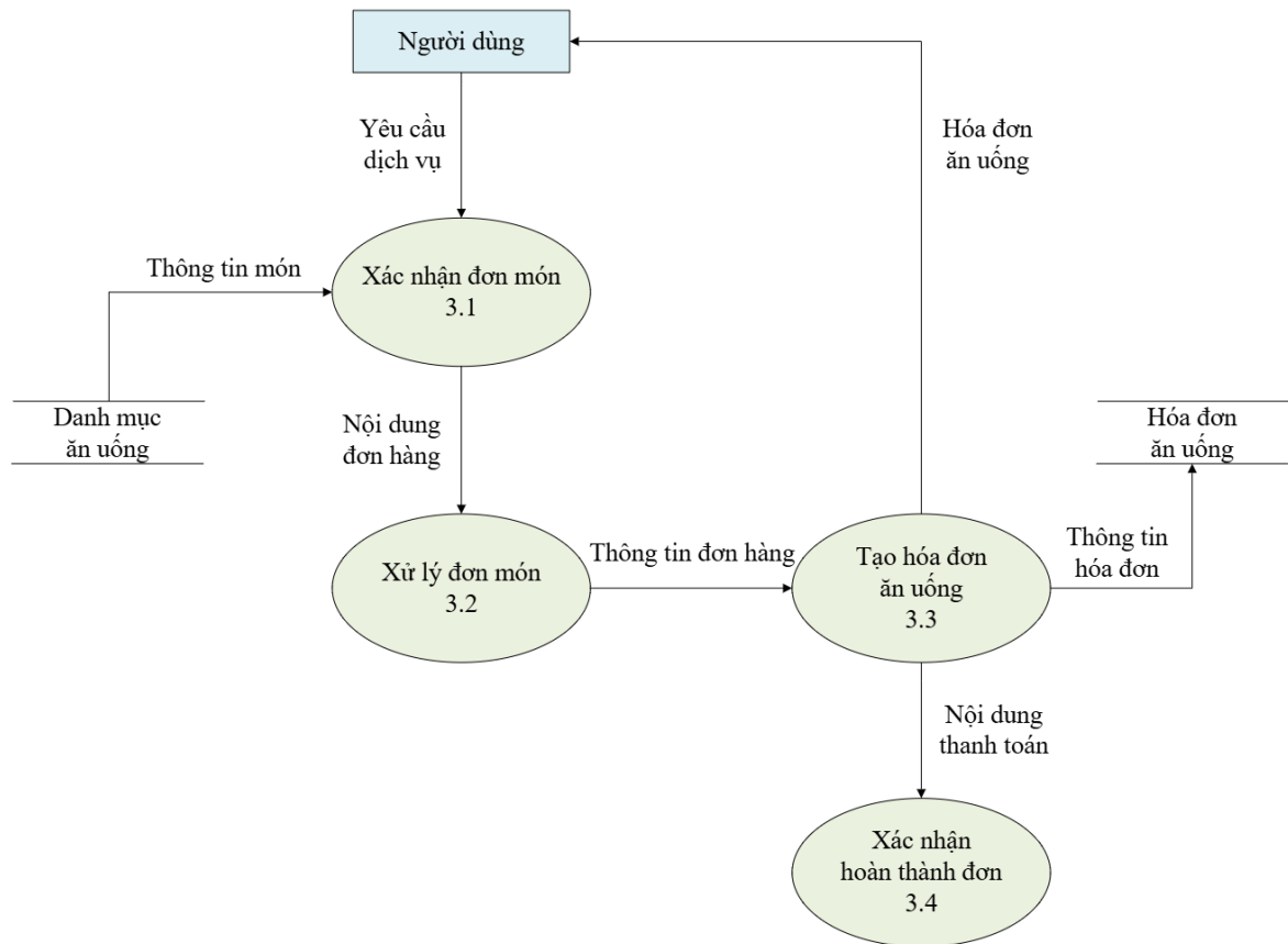
Hình 3.6: Sơ đồ DFD mức 1 - Xử lý dịch vụ ăn uống
