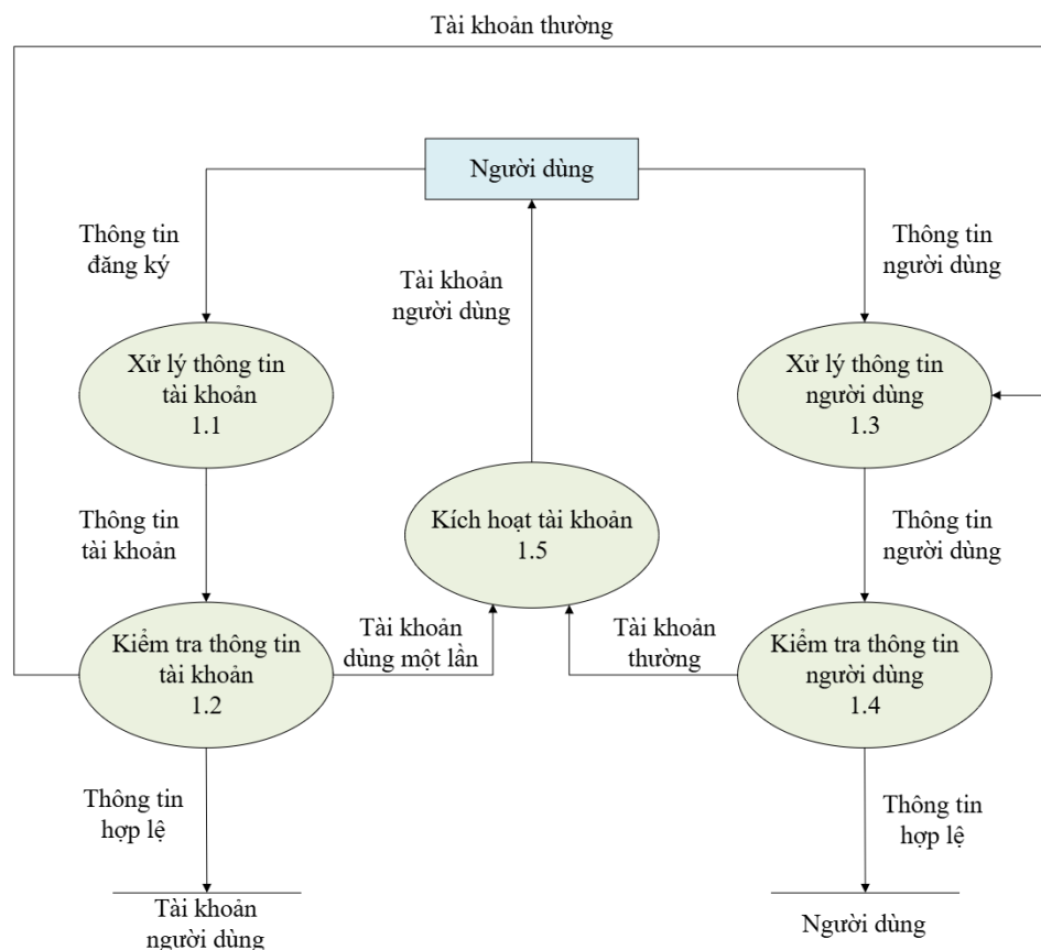
Hình 3.4: Sơ đồ DFD mức 1 - đăng ký tài khoản
