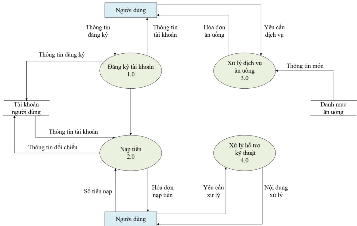
Hình 3.3: Sơ đồ DFD mức 0
