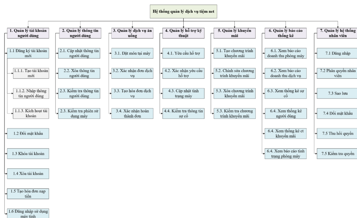
Hình 3.1: Mô hình phân cấp chức năng (BFD)
