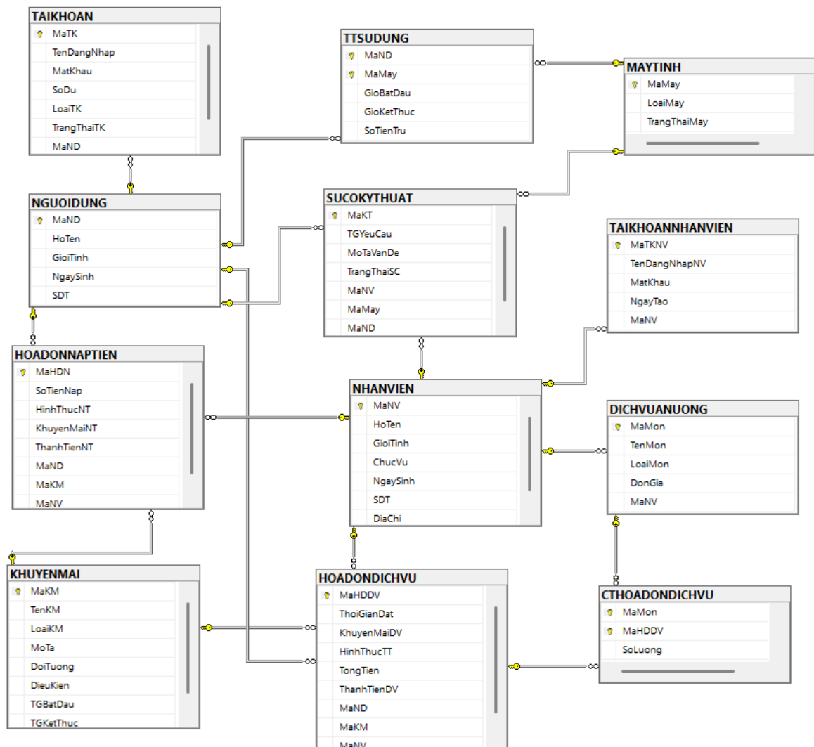
Hình 3.11: Database diagram
