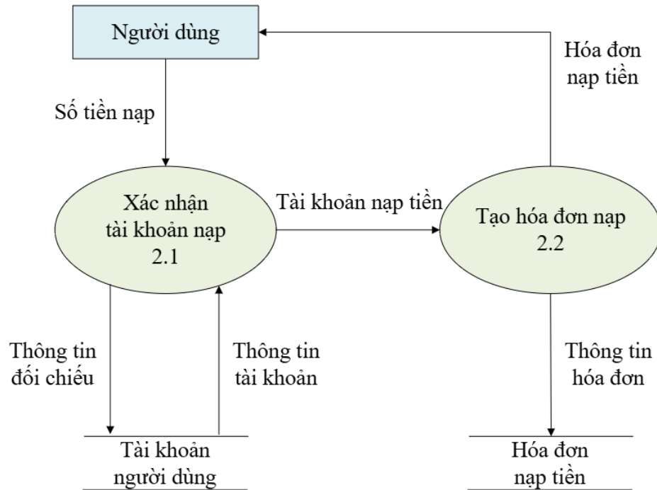
Hình 3.5: Sơ đồ DFD mức 1 - nạp tiền
