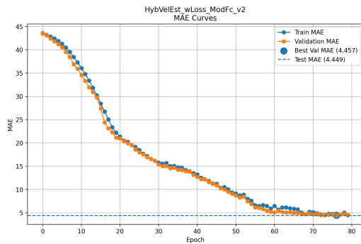
Figura 8: Curvas de aprendizaje del Error Absoluto Medio (MAE) para HybridVelocityEstimator.
