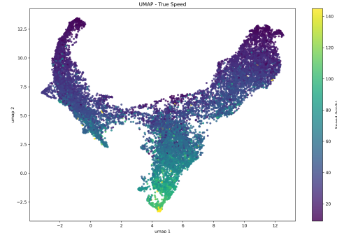
Figura 5: Visualización bidimensional de los embeddings generados por el modelo ImageVelocityEstimator.
