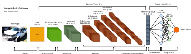
Figura 2: Arquitectura de ImageVelocityEstimator.
