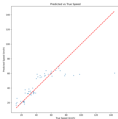
Figura 17: Diagrama de dispersión entre velocidades predichas y velocidades reales para el modelo XGBoost entrenado con el Pipeline de Preprocesamiento 3
