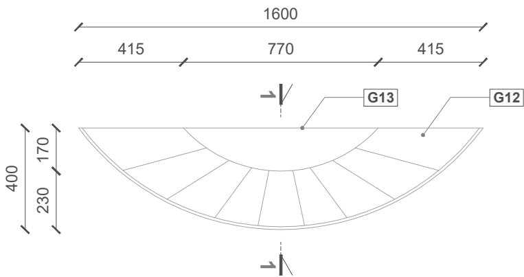
1 MẶT BỀ
