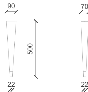
G11 - MẶT ĐỨNG G11 - MẶT BÊN
