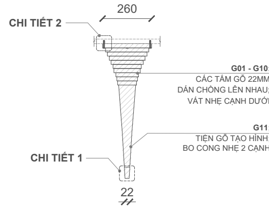
8 CHÂN BÀN - MẶT CẮT 2
