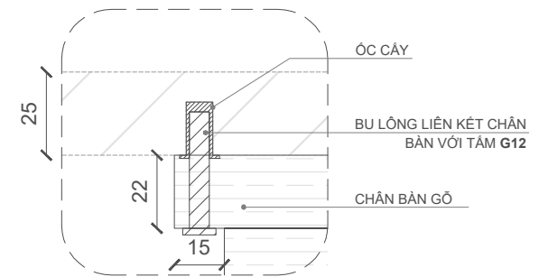
9 CHI TIẾT 2 - LIÊN KẾT CHÂN BÀN VÀ MẶT BÀN
