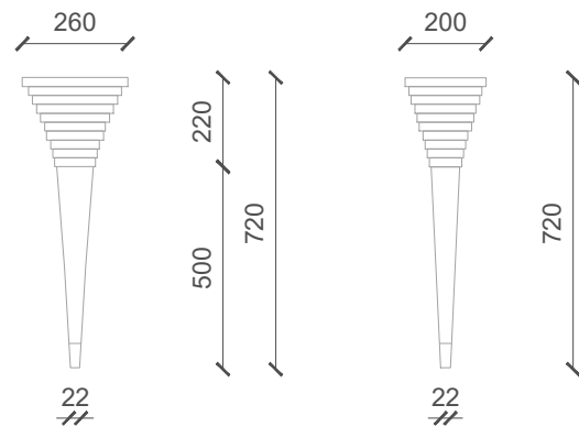
7 CHÂN BÀN - MẶT ĐỨNG & MẶT BÊN
