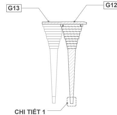
4 MẶT CẮT 1
