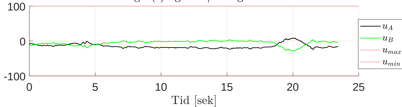
Pådrag u(t) og max/min-grensene.
