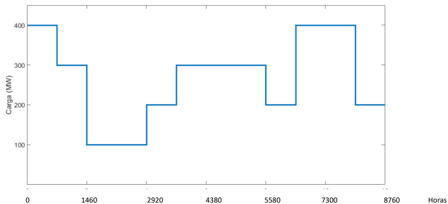
Curva de Carga Anual
