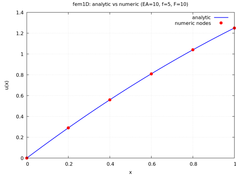
Figure 1: So sánh nghiệm analytic và các im nút nghiệm s ( EA=10 , f = 5 , F = 10 ).
