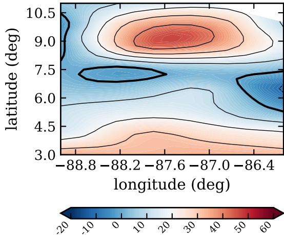
RF01, day 219, dcin, (J/K/kg)
