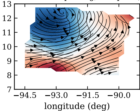
BL winds 20 m/s per deg, surf pres (hPa)
