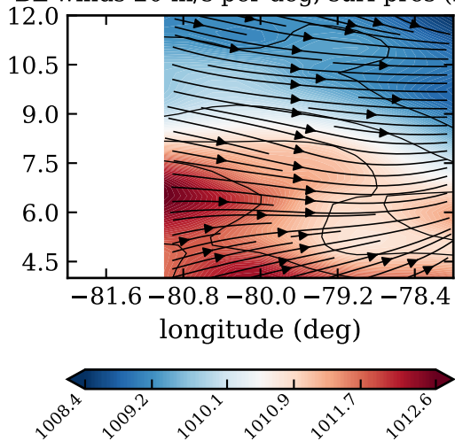
BL winds 20 m/s per deg, surf pres (hPa)
