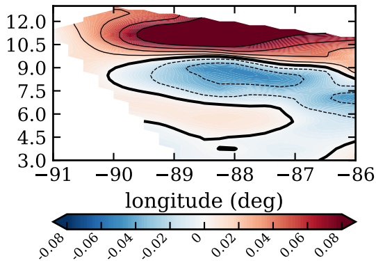
RF14, day 264, mfluxdif (kg/m 2 /s)
