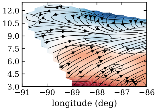
BL winds 20 m/s per deg, surf pres (hPa)
