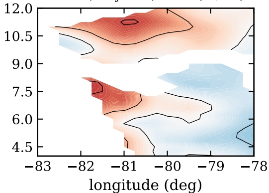
RF15c, day 265, eflux (W/m 2 )
