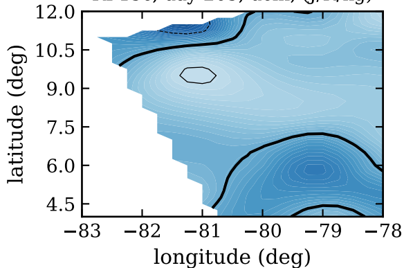
RF15c, day 265, dcin, (J/K/kg)
