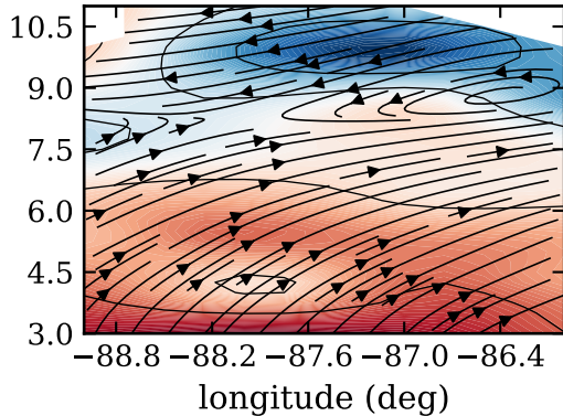
BL winds 20 m/s per deg, surf pres (hPa)
