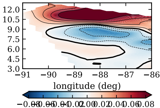
RF14, day 264, mfluxdif (kg/m 2 /s)
