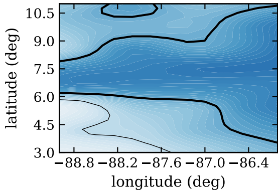
RF21, day 274, dcin, (J/K/kg)
