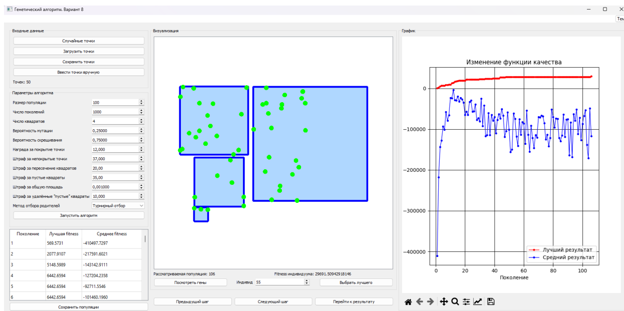
Рисунок 11 – Пример успешного завершения алгоритма с 50 точками
