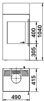
GALILEO Acier 2 côtés
