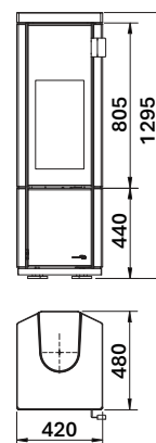
CONTE mini droit
