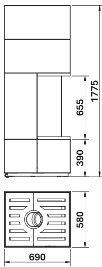
LINEA KLG Gaz
