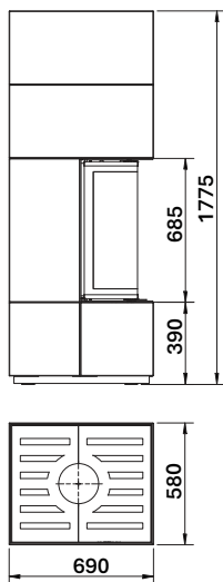
LINEA KL1 Béton
