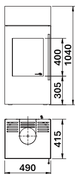
GALILEO Acier 3 côtés
