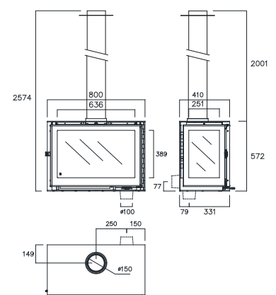
Laria 80 LI + T
