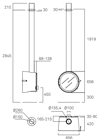
A4520 Pied en option.
