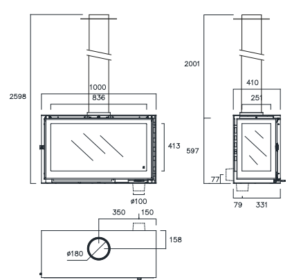
Laria 100 LI + T
