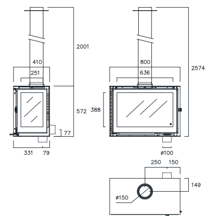
Laria 80 LD + T
