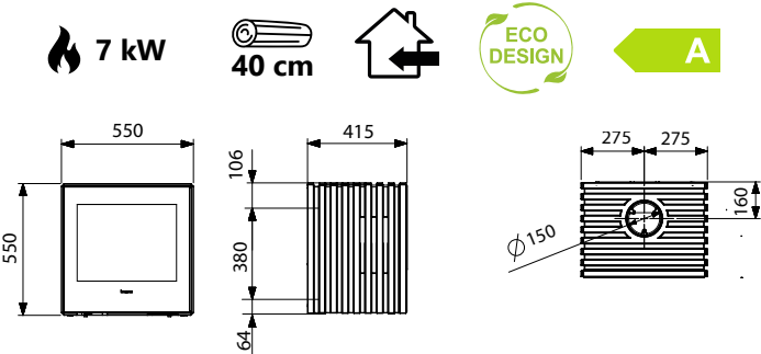
GLANCE MWB - MURAL OU SUR BANC
