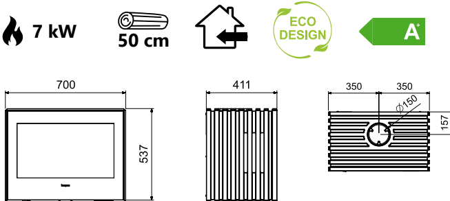
GLANCE LWB - MURAL OU SUR BANC
