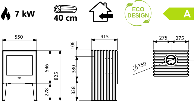
GLANCE M - SUR PIEDS
