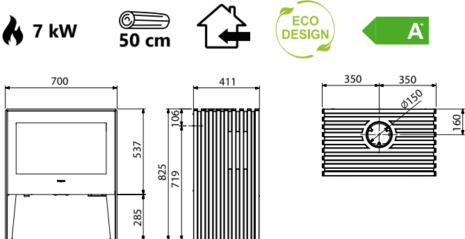
GLANCE L - SUR PIEDS
