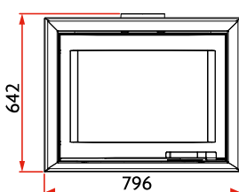
XP68 BOX MODUL'air CUBE
