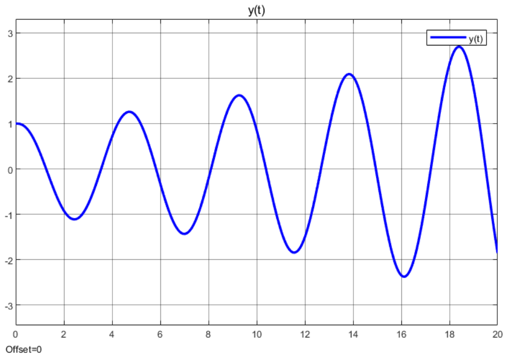
Рис. 14: K = 10, T_1 = 5, T_2 = \frac{1}{6} неустойчивая система
