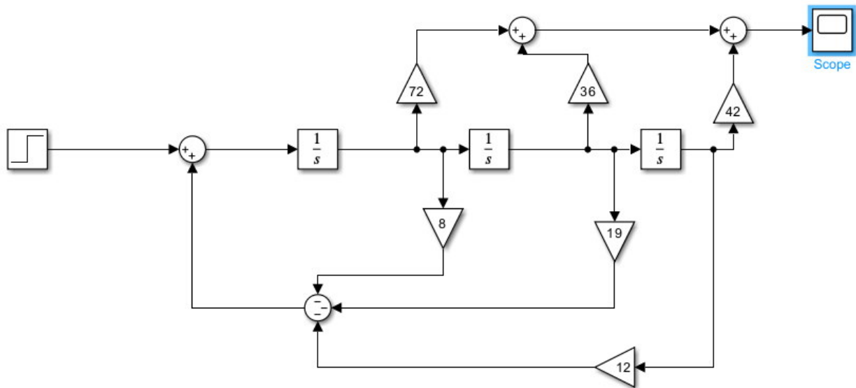
Рис. 1: Схема моделирования задания 1
