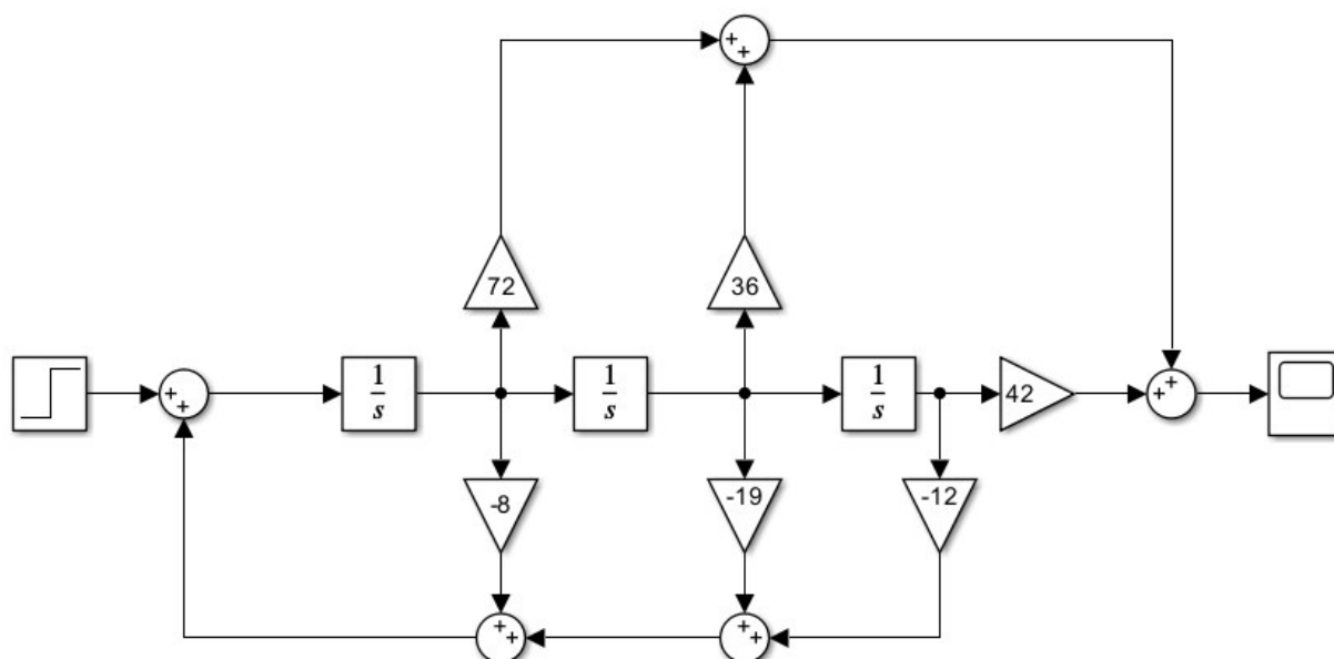
Рис. 7: Схема моделирования системы в канонической управляемой форме
