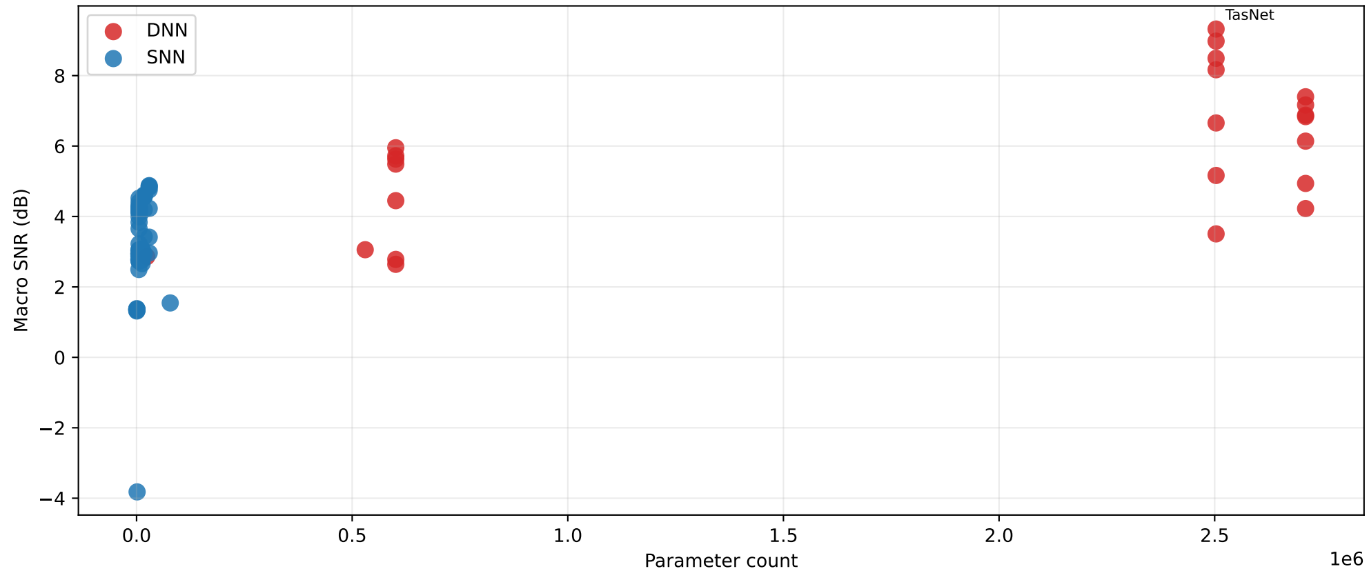
Macro SNR vs parameter count
